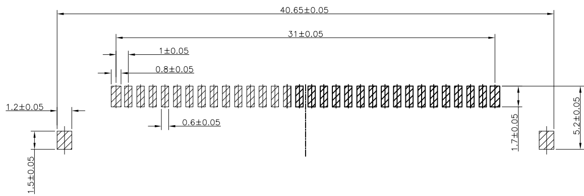
P.C.B LAYOUT SCAL 1:1
