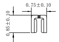
d-d section
