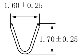
a-a section
