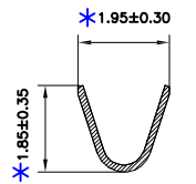
SECTION A-A SCALE 1:1
