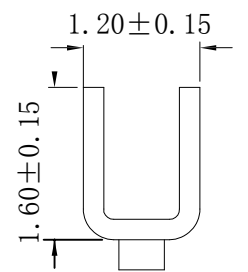
SEC:C--C
